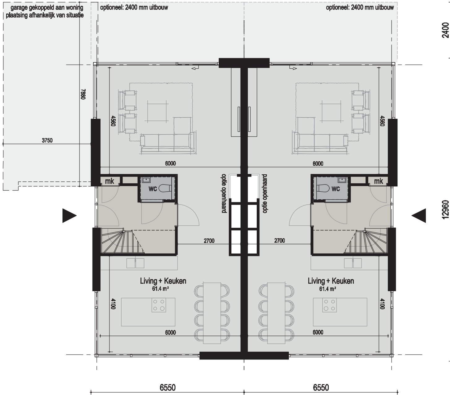
BEGANE GROND bouwnummer 17
