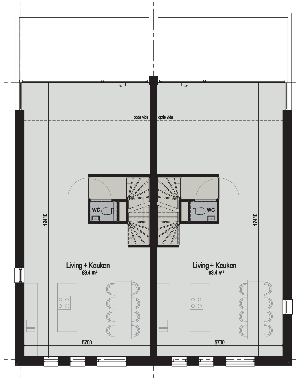
EERSTE VERDIEPING bouwnummers 20 en 22
